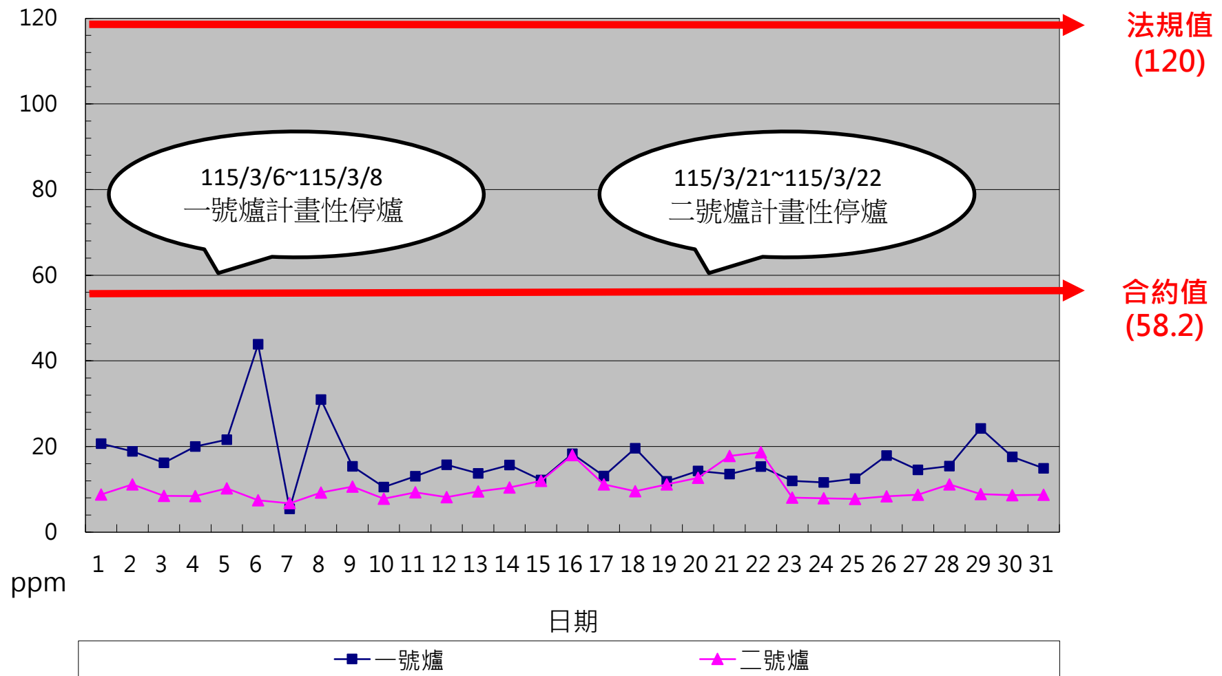
一百一十五年三月份 CO單日24小時平均整月排放監測紀錄
