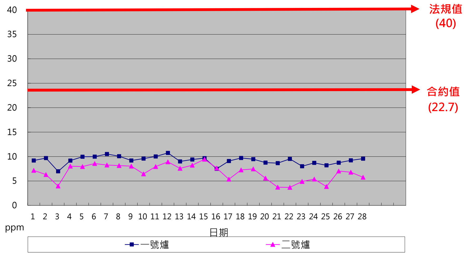
一百一十五年二月份 HCl單日24小時整月排放監測紀錄
