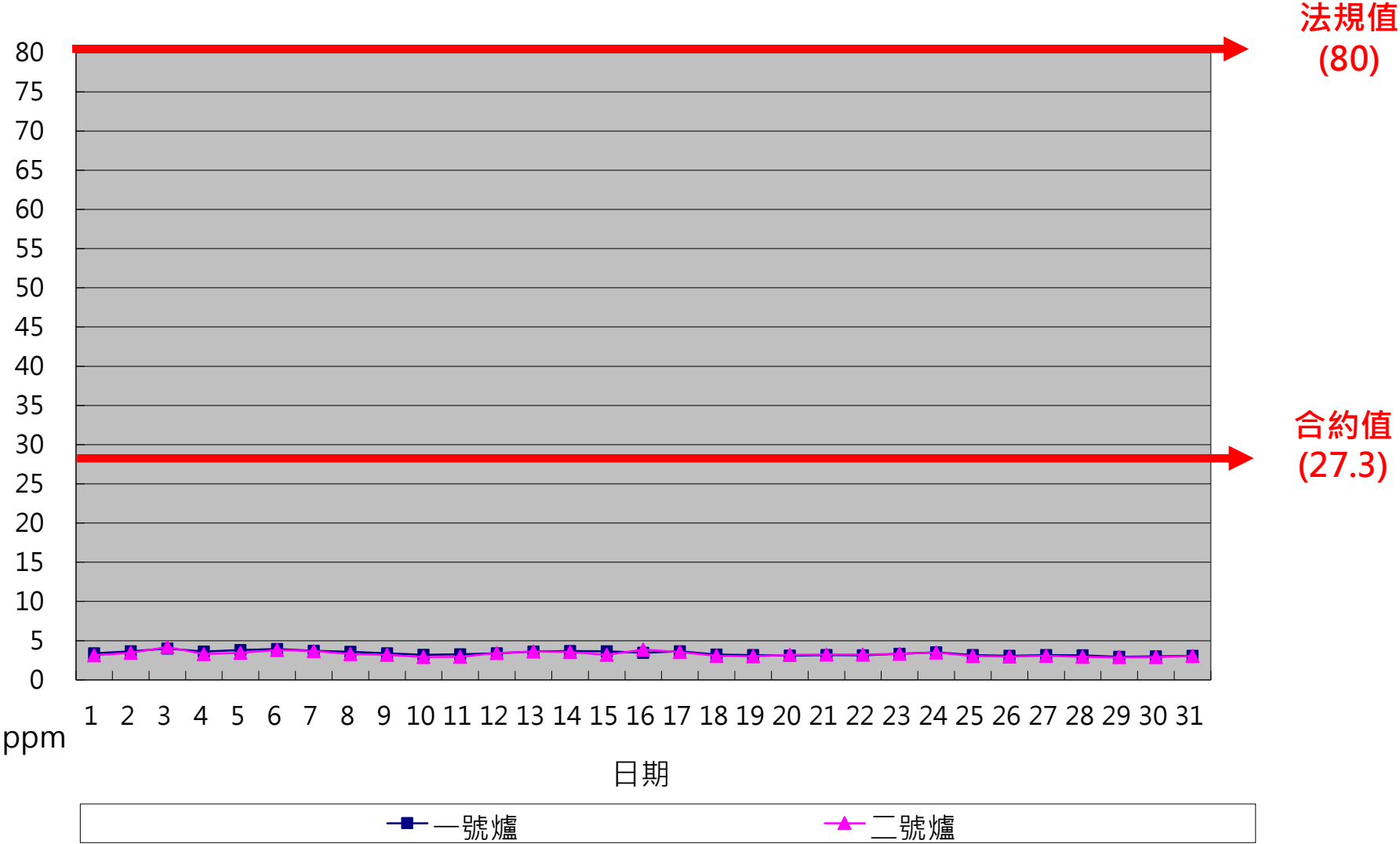
一百一十四年七月份 SO x 單日24小時整月排放監測紀錄
