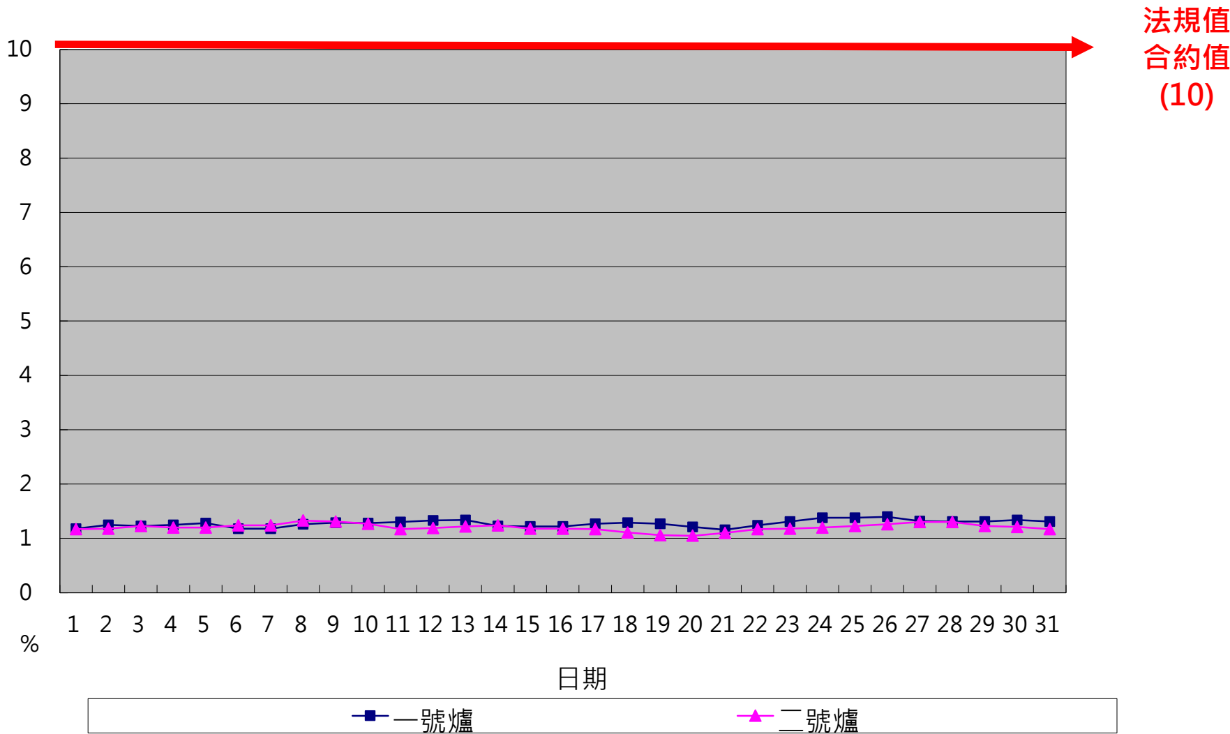
一百一十四年七月份 OPACITY單日24小時整月排放監測紀錄
