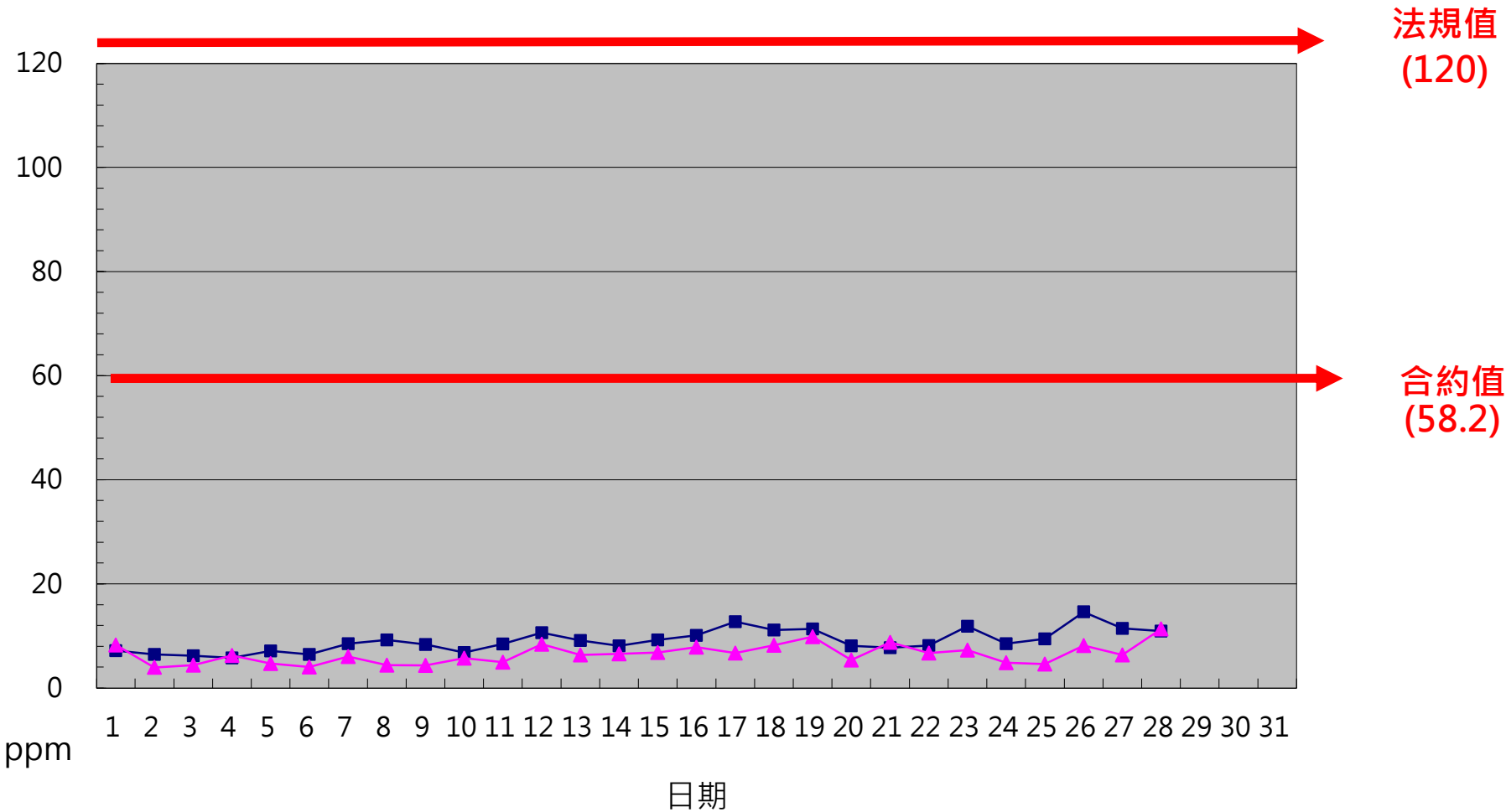
一百一十四年二月份 CO單日24小時平均整月排放監測紀錄
