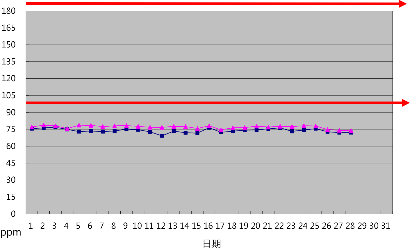
一百一十四年二月份 NO x 單日24小時整月排放監測紀錄
