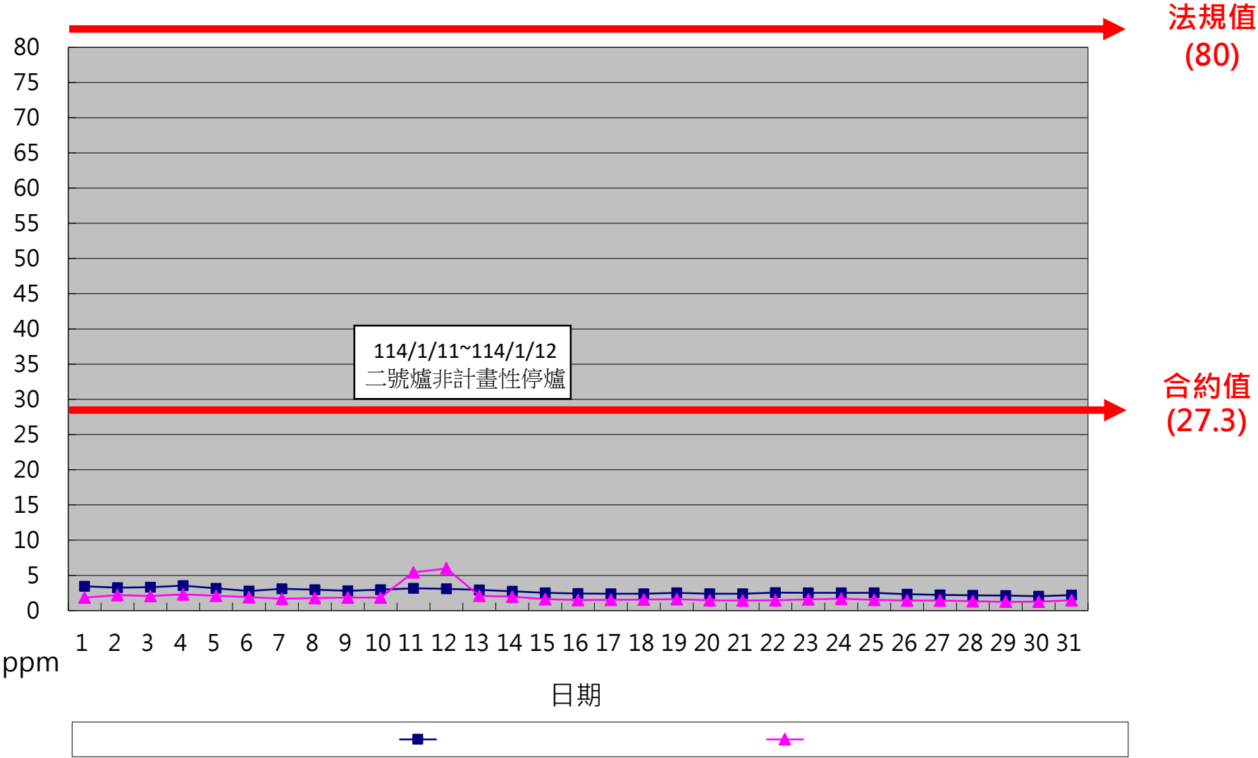
一百一十四年一月份 SO x 單日24小時整月排放監測紀錄
