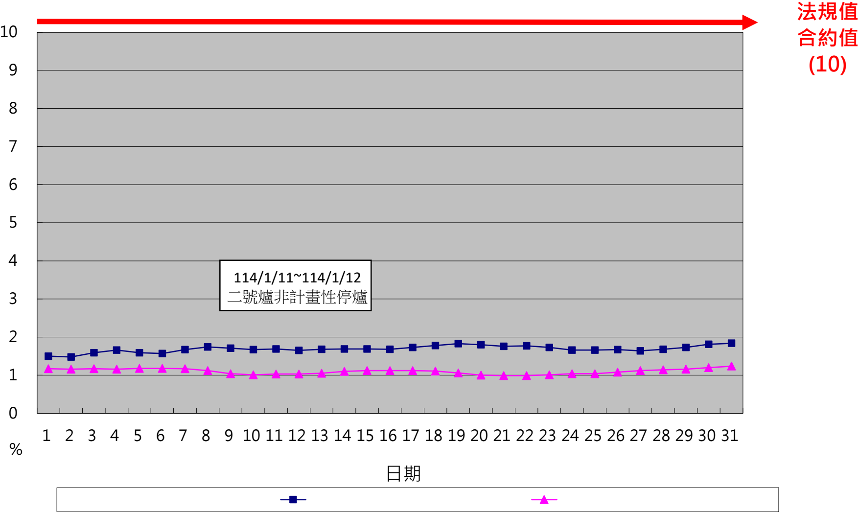
一百一十四年一月份 OPACITY單日24小時整月排放監測紀錄
