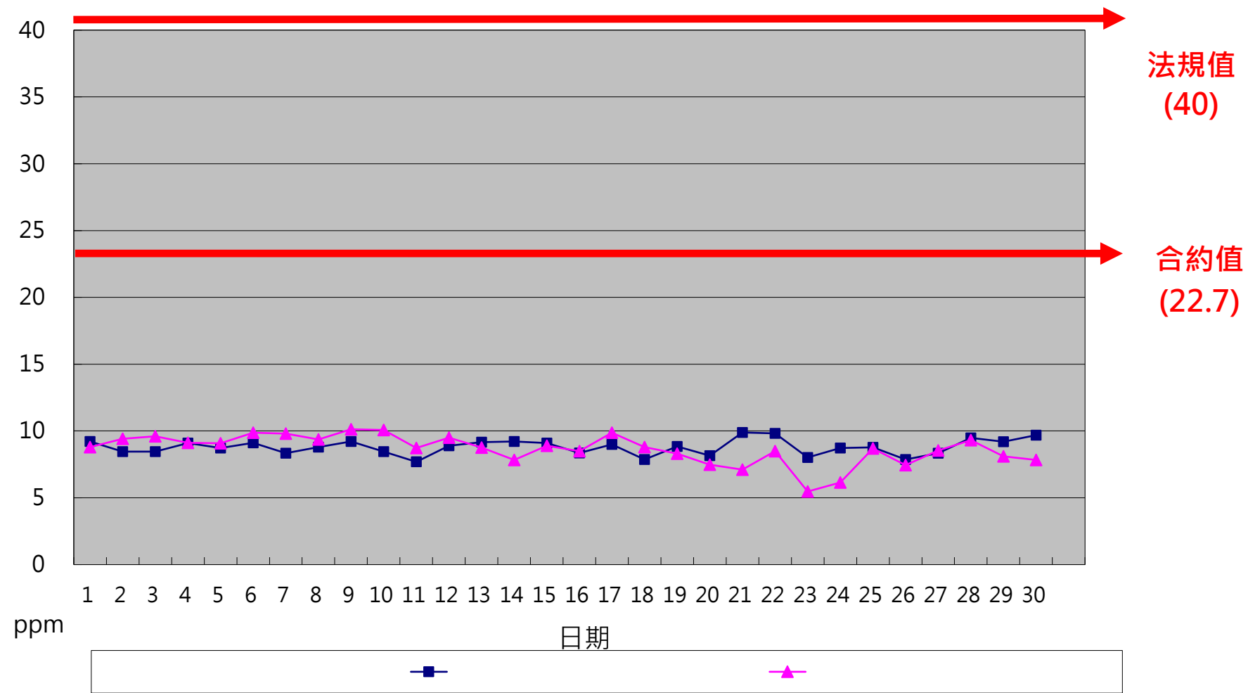
一百一十三年九月份 HCl單日24小時整月排放監測紀錄
