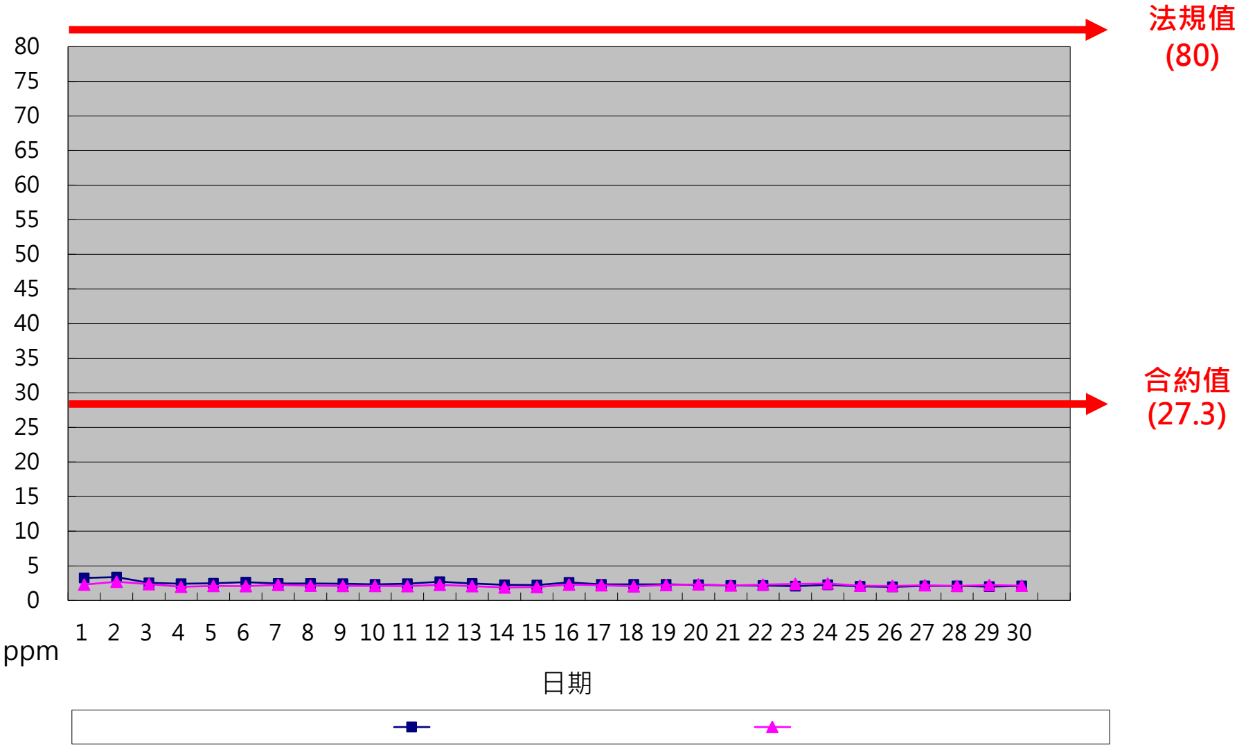
一百一十三年九月份 SO x 單日24小時整月排放監測紀錄
