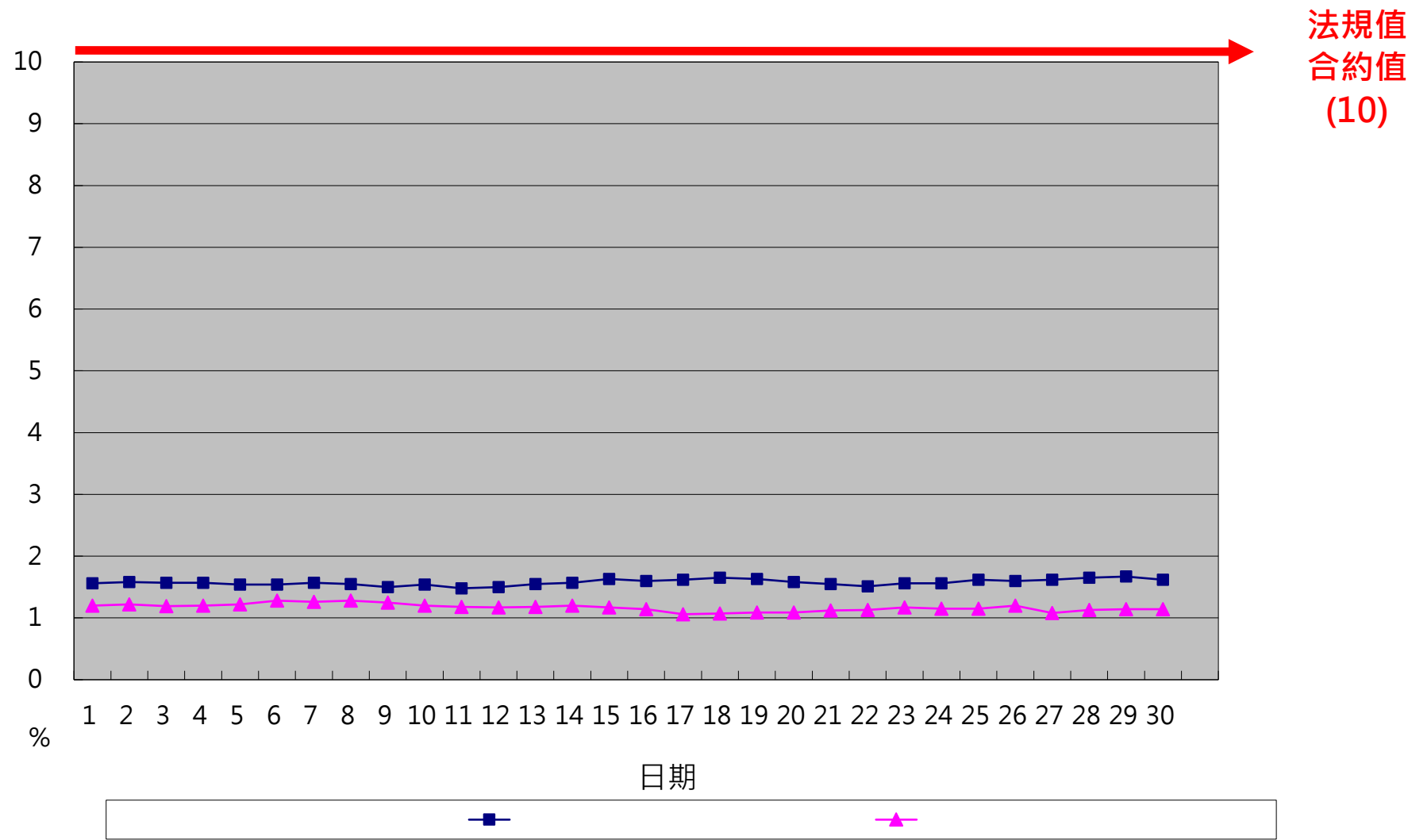
一百一十三年九月份 OPACITY單日24小時整月排放監測紀錄
