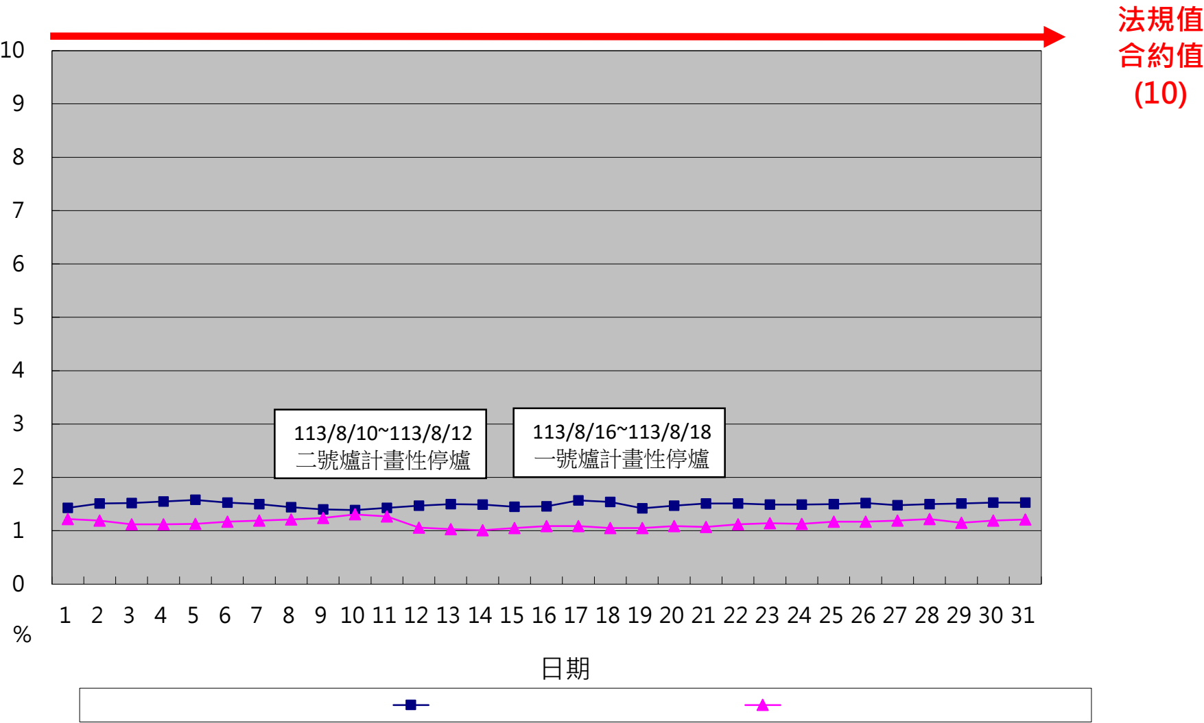
一百一十三年八月份 OPACITY單日24小時整月排放監測紀錄
