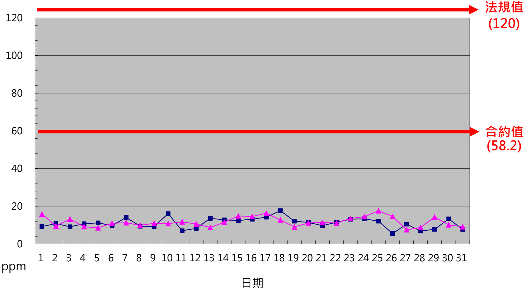
一百一十三年七月份 CO單日24小時平均整月排放監測紀錄
