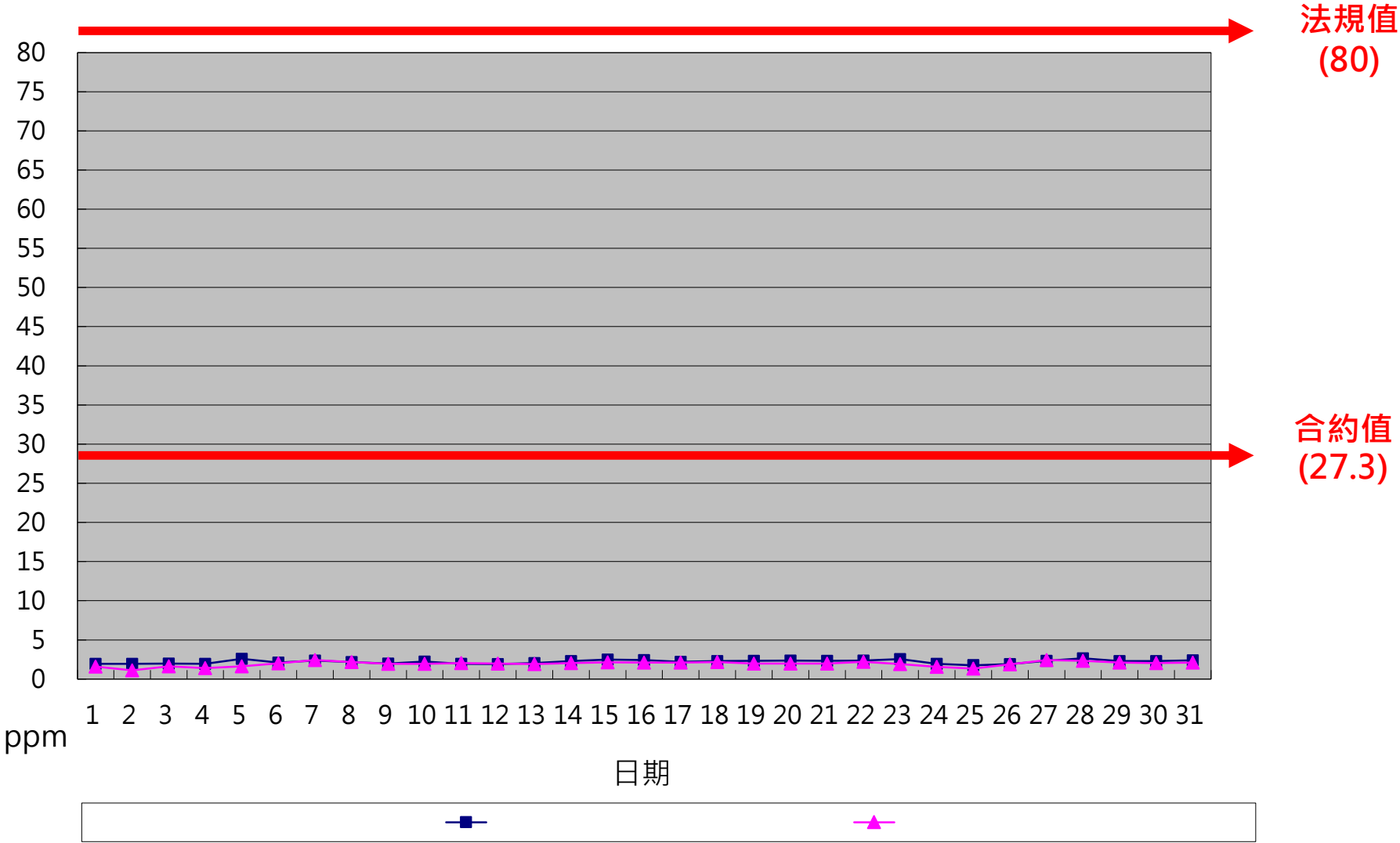
一百一十三年七月份 SO x 單日24小時整月排放監測紀錄
