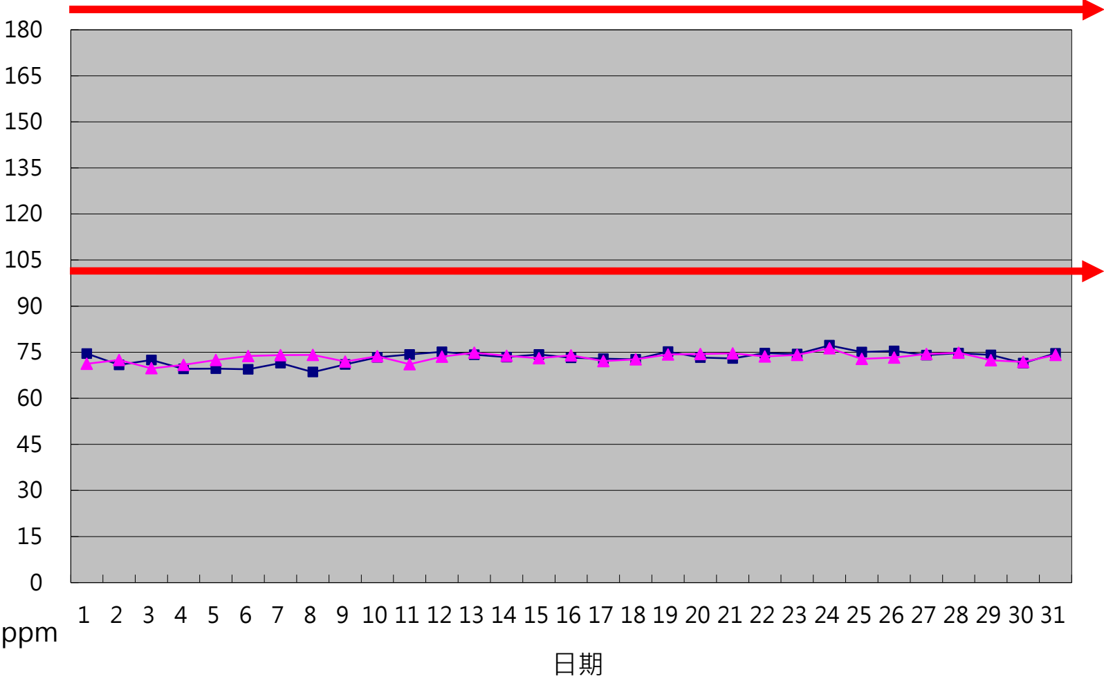
一百一十三年七月份 NO x 單日24小時整月排放監測紀錄
