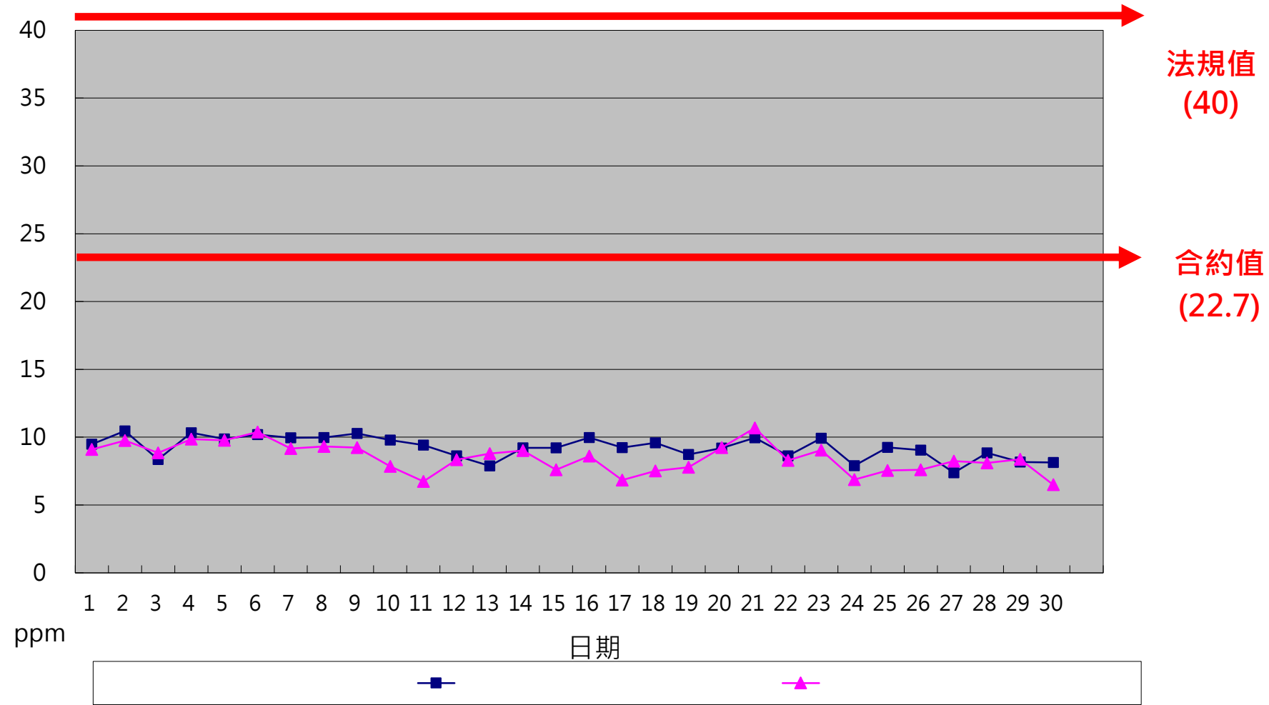
一百一十三年六月份 HCl單日24小時整月排放監測紀錄
