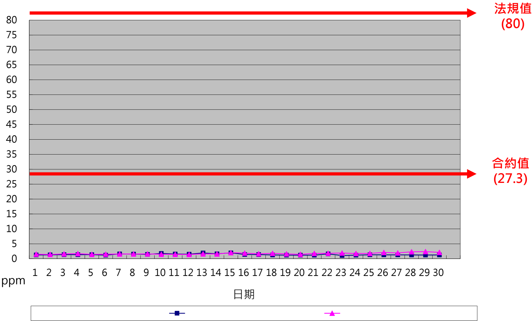
一百一十三年四月份 SO x 單日24小時整月排放監測紀錄
