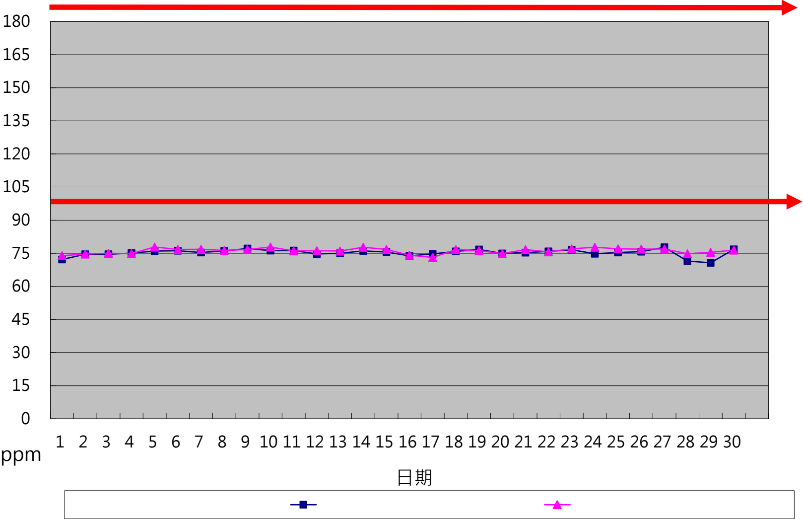
一百一十三年四月份 NO x 單日24小時整月排放監測紀錄
