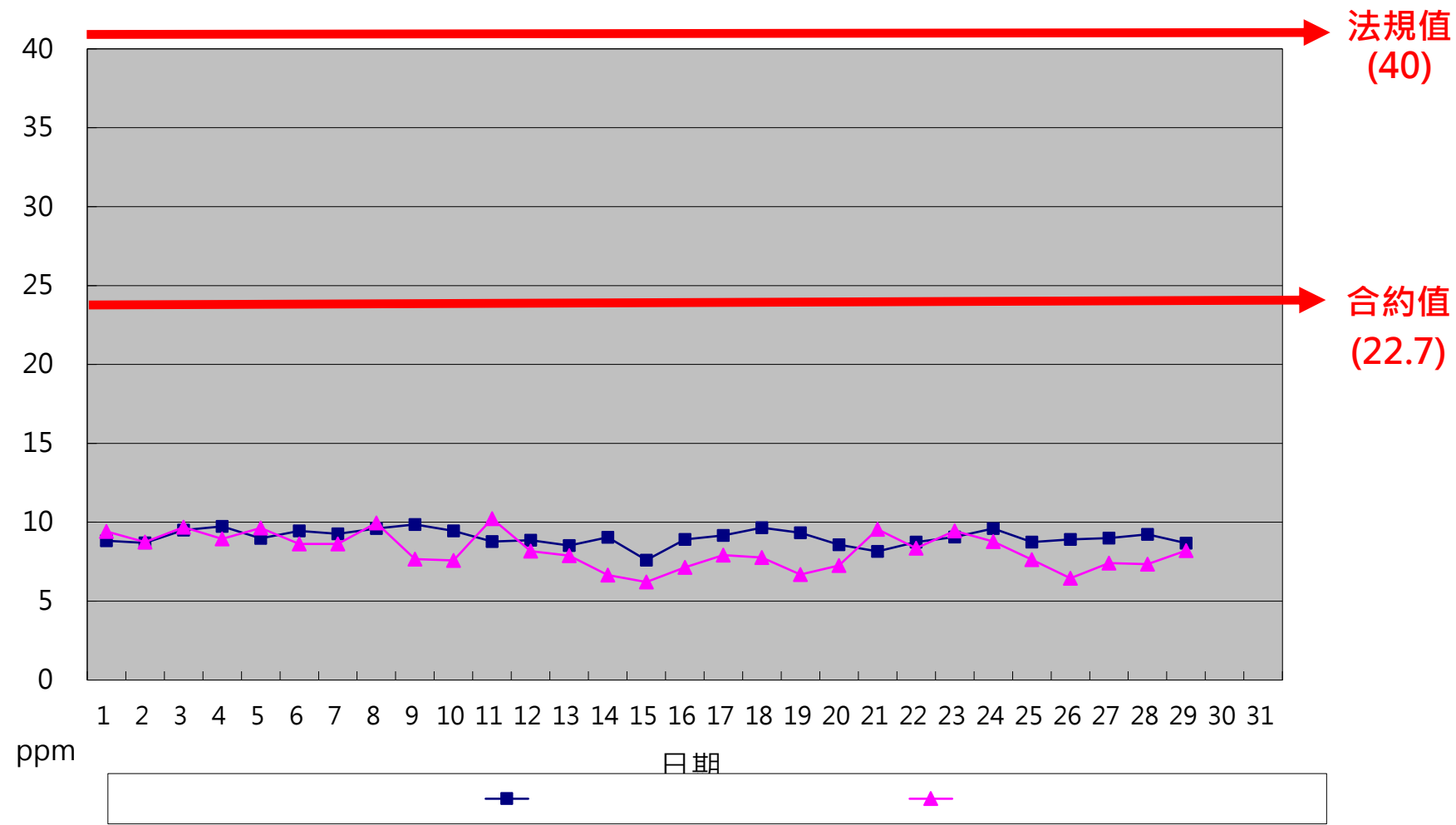
一百一十三年二月份 HCl單日24小時整月排放監測紀錄
