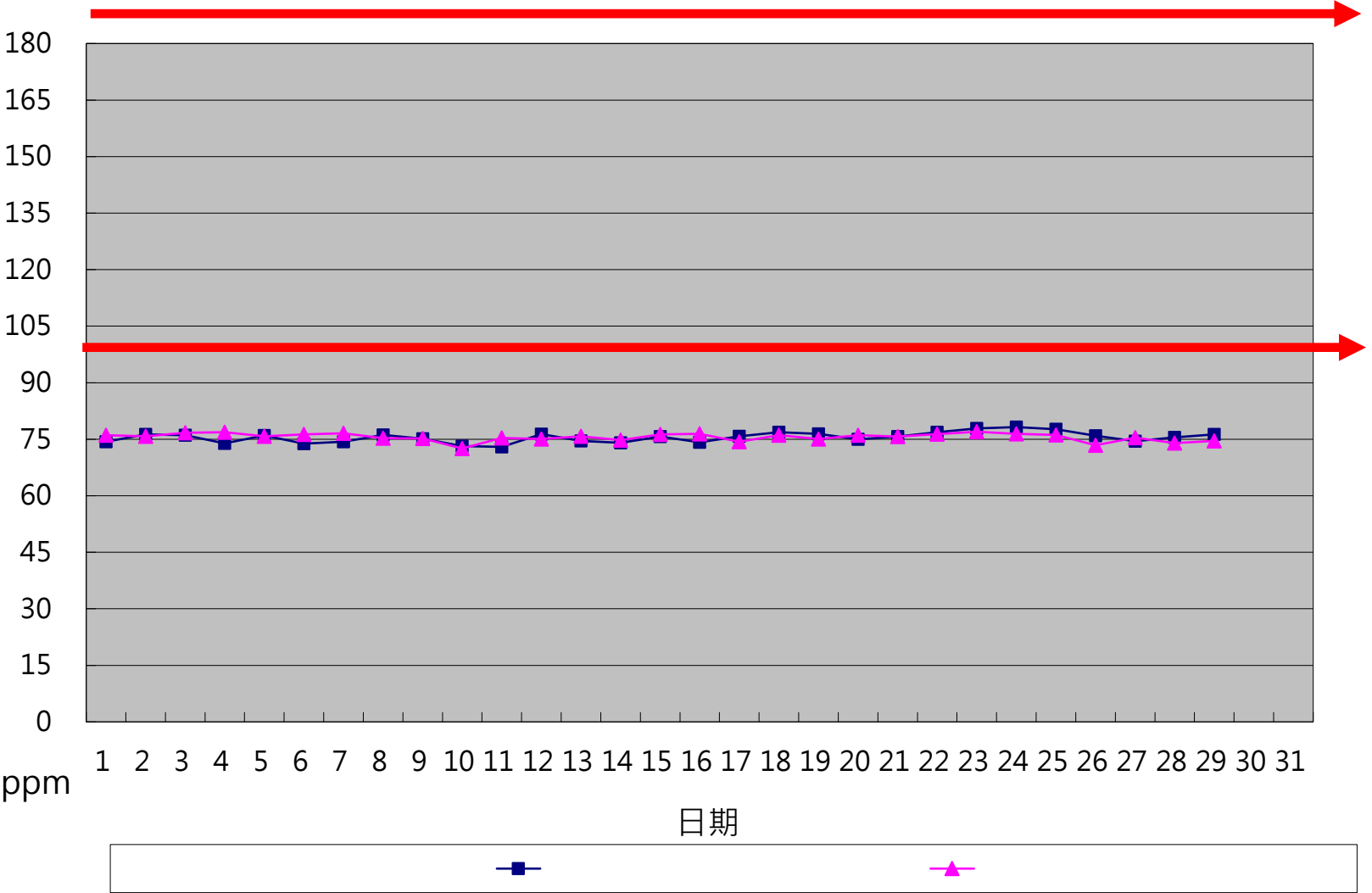
一百一十三年二月份 NO x 單日24小時整月排放監測紀錄
