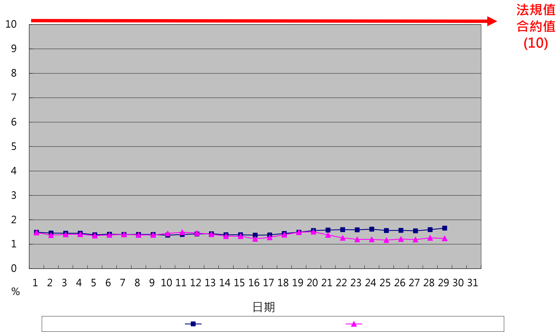
一百一十三年二月份 OPACITY單日24小時整月排放監測紀錄
