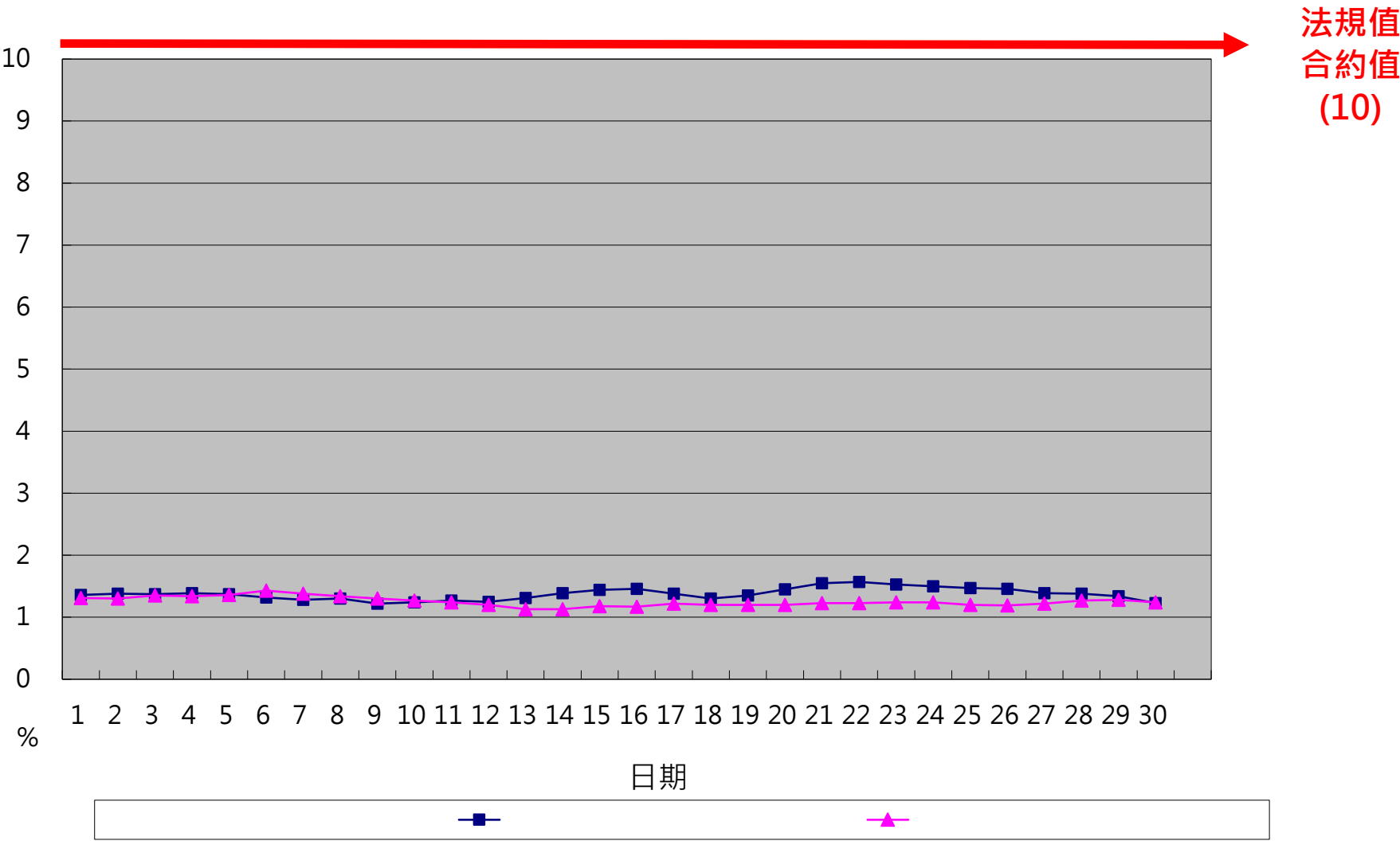
一百一十二年十一月份 OPACITY單日24小時整月排放監測紀錄
