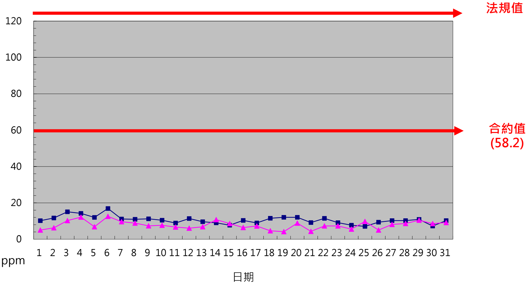
一百一十二年七月份 CO單日24小時平均整月排放監測紀錄
