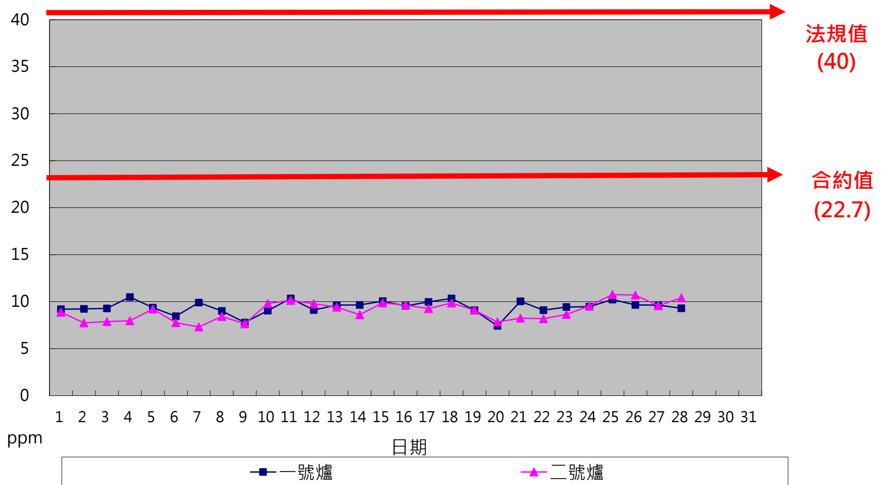
一百一十二年二月份 HCl單日24小時整月排放監測紀錄
