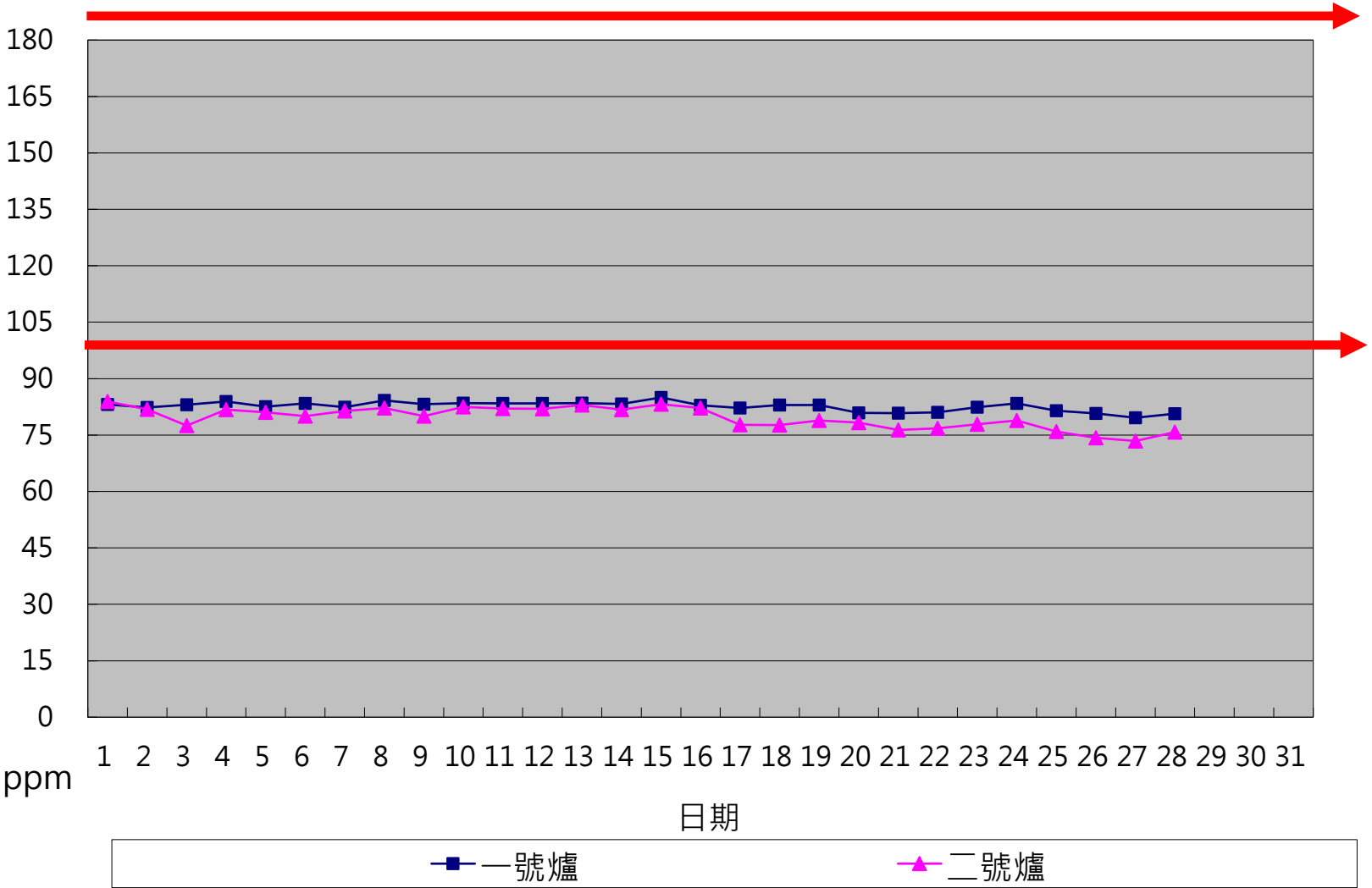
一百一十二年二月份 NO x 單日24小時整月排放監測紀錄
