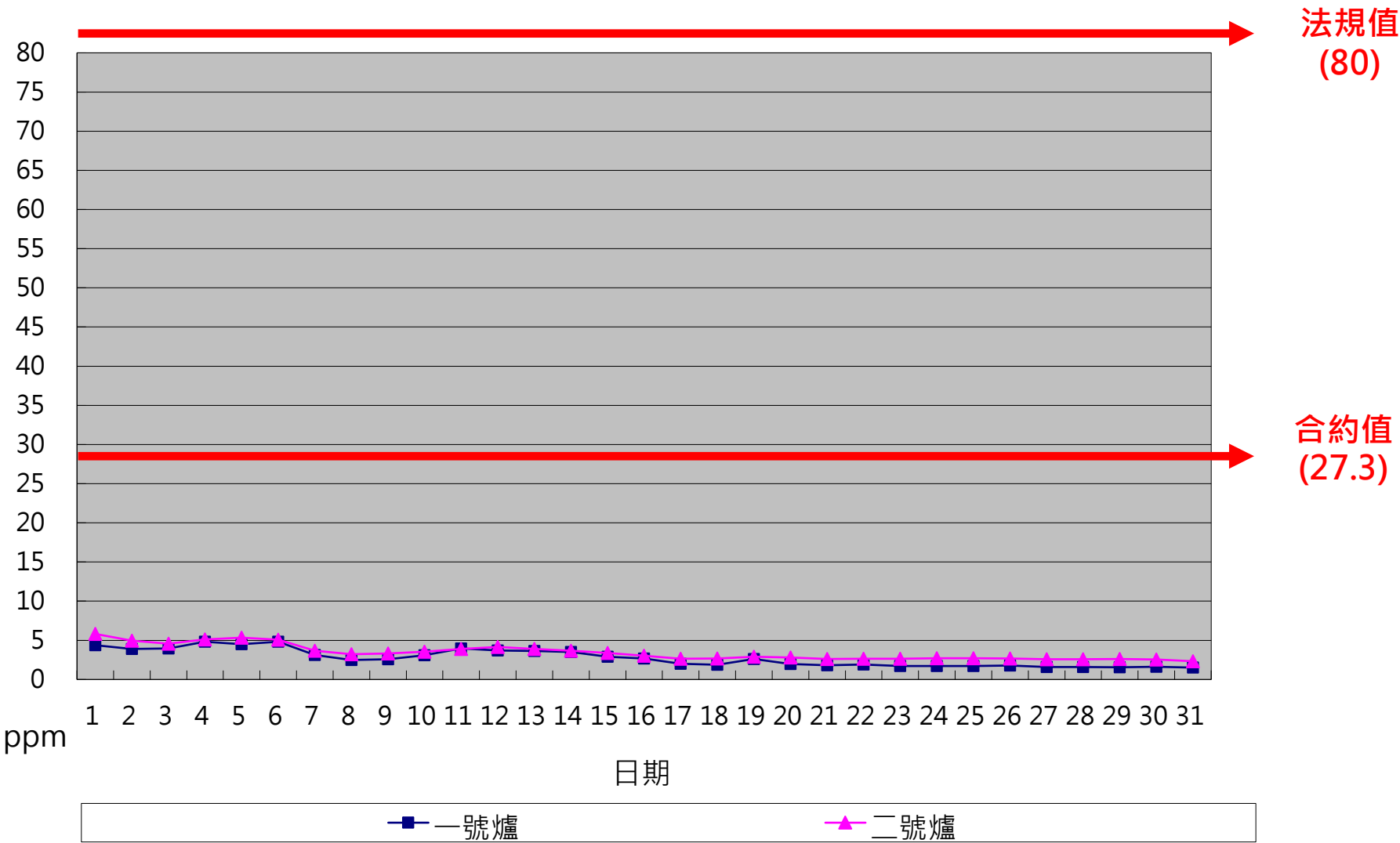
一百一十二年一月份 SO x 單日24小時整月排放監測紀錄
