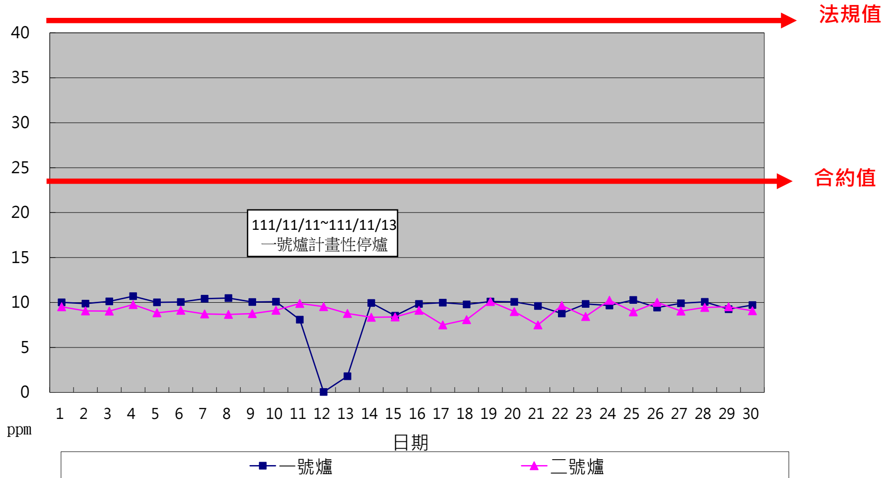
一百一十一年十一月份 HCl單日24小時整月排放監測紀錄
