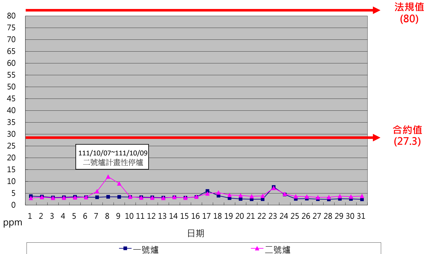
一百一十一年十月份 \text{SO}_x 單日24小時整月排放監測紀錄
