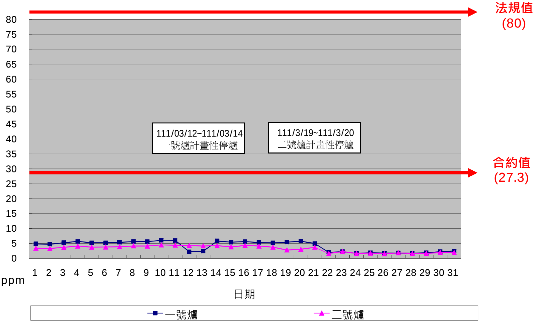
一百一十一年三月份 SO x 單日24小時整月排放監測紀錄
