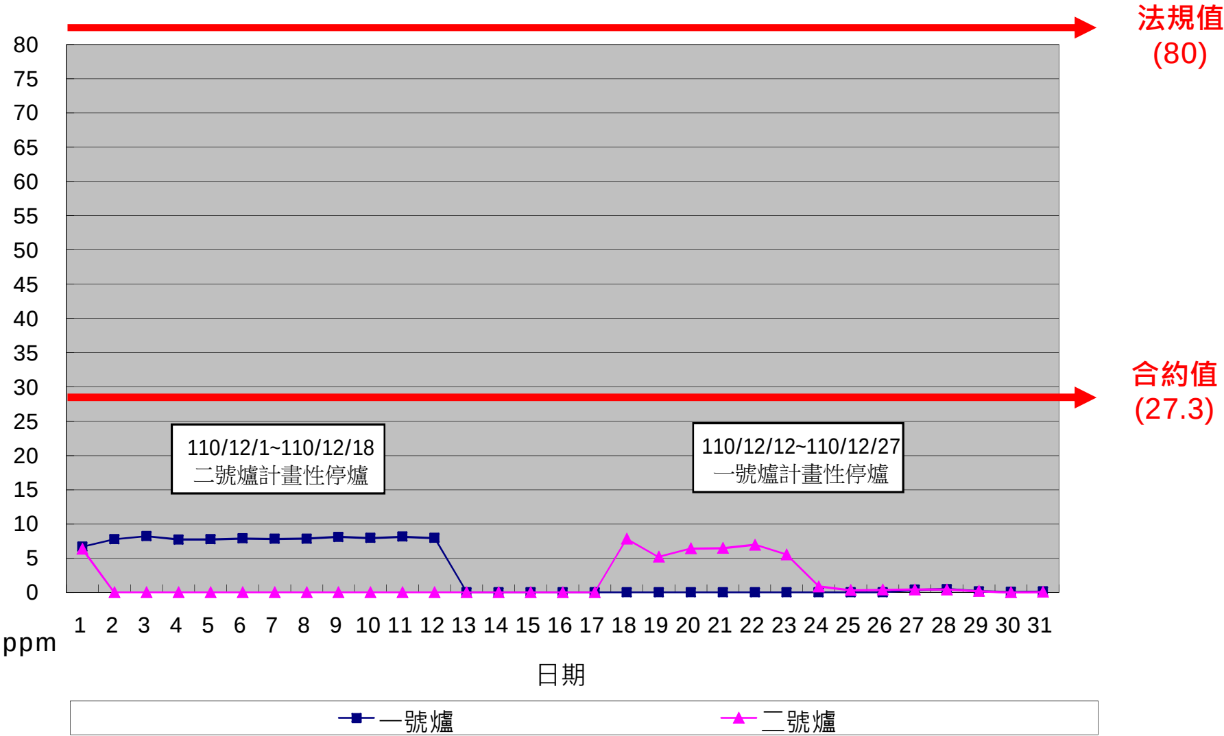
一百一十年十二月份 SO x 單日24小時整月排放監測紀錄
