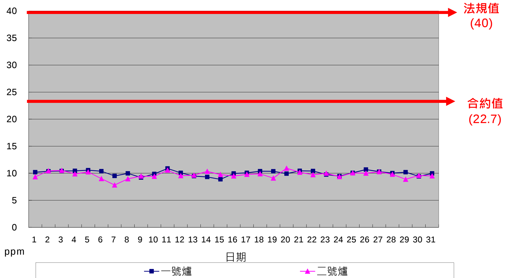
一百一十年七月份 HCl單日24小時整月排放監測紀錄
