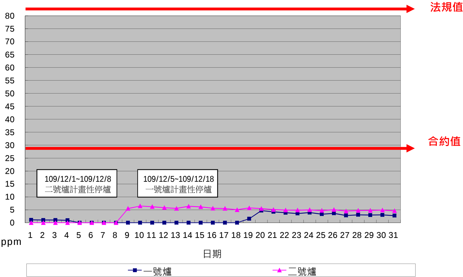
一百零九年十二月份 SO x 單日24小時整月排放監測紀錄
