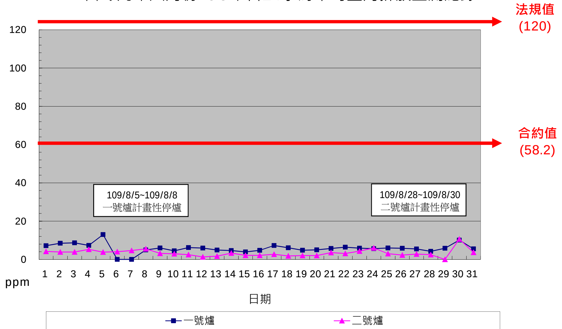
一百零九年八月份 CO單日24小時平均整月排放監測紀錄
