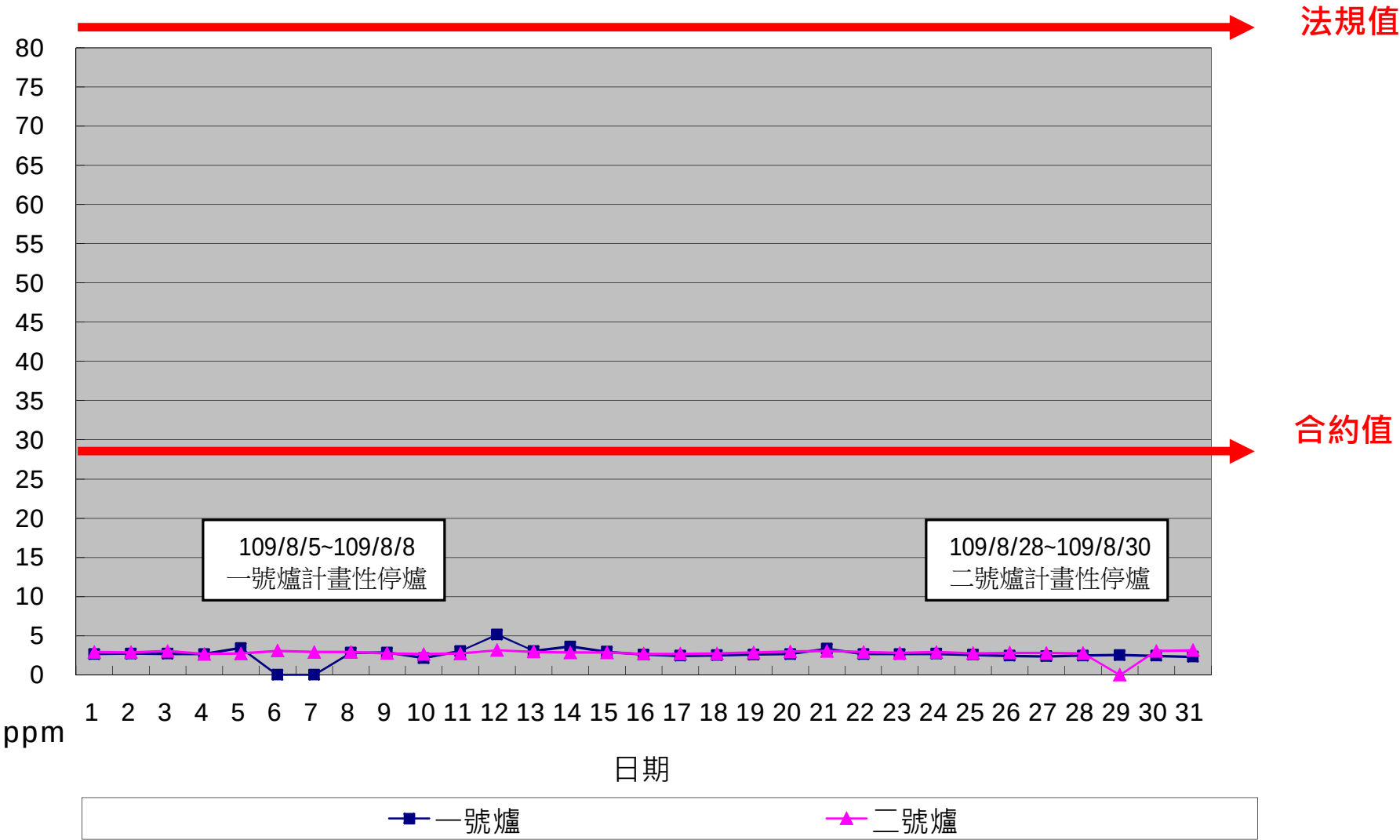
一百零九年八月份 SO x 單日24小時整月排放監測紀錄
