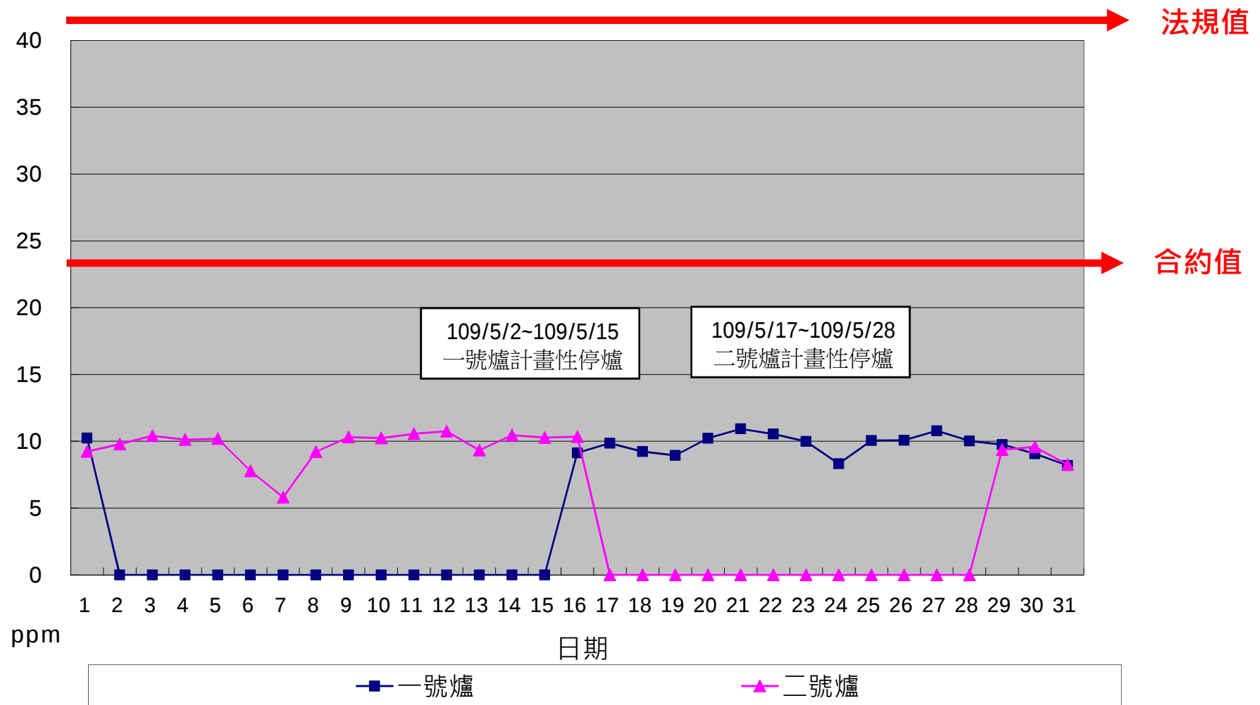
一百零九年五月份 HCl單日24小時整月排放監測紀錄
