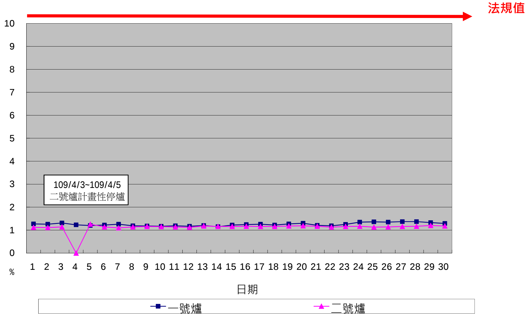
一百零九年四月份 OPACITY單日24小時整月排放監測紀錄
