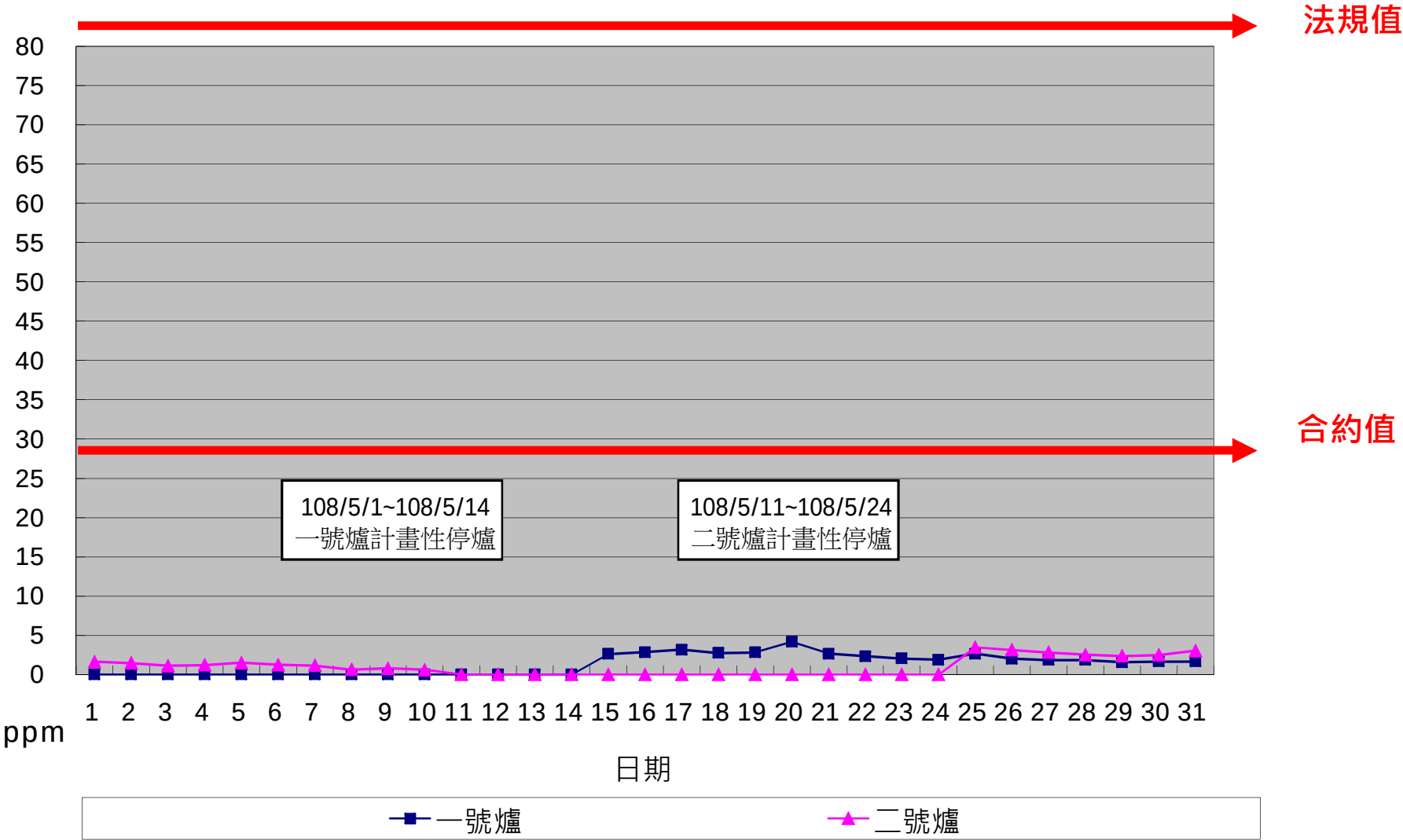
一百零八年五月份 SO x 單日24小時整月排放監測紀錄
