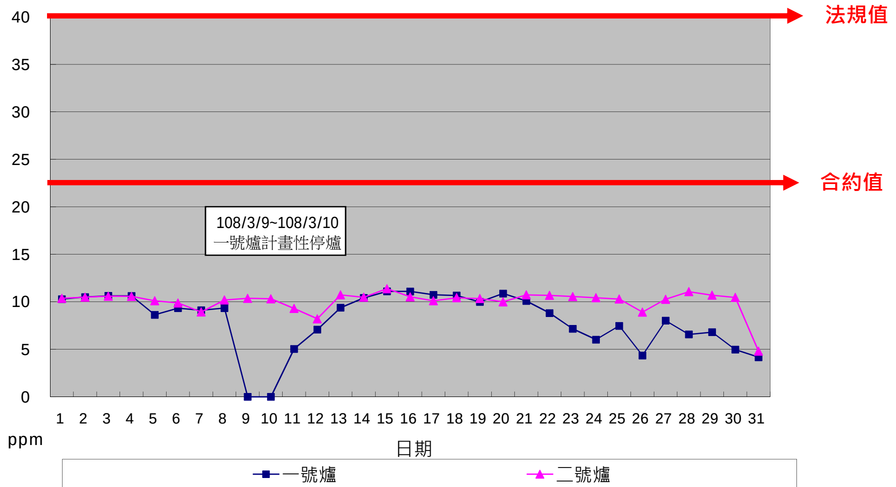
一百零八年三月份 HCl單日24小時整月排放監測紀錄
