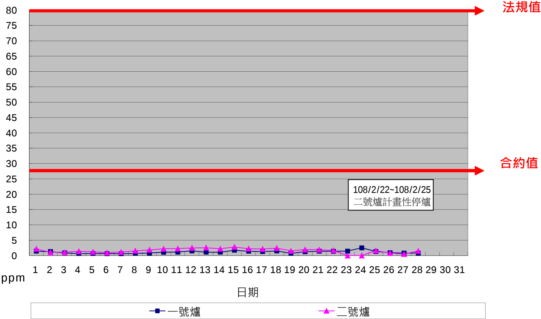
一百零八年二月份 SO x 單日24小時整月排放監測紀錄
