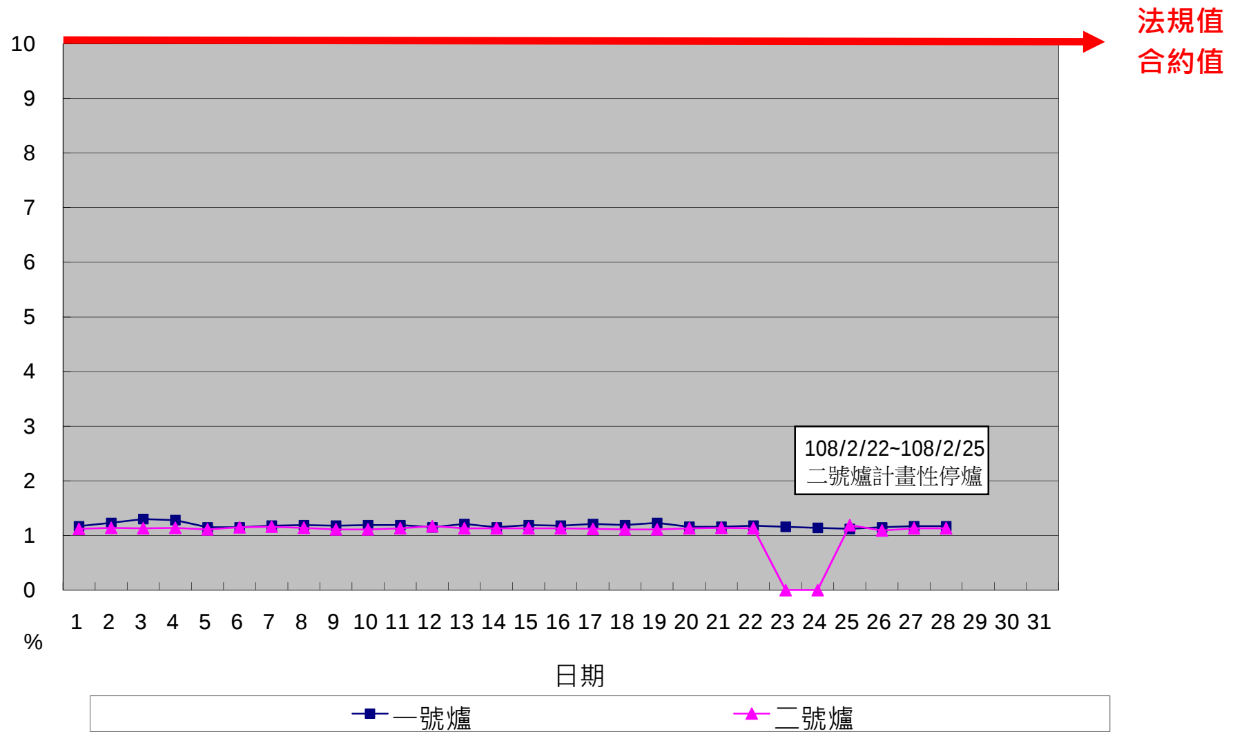
一百零八年二月份 OPACITY單日24小時整月排放監測紀錄
