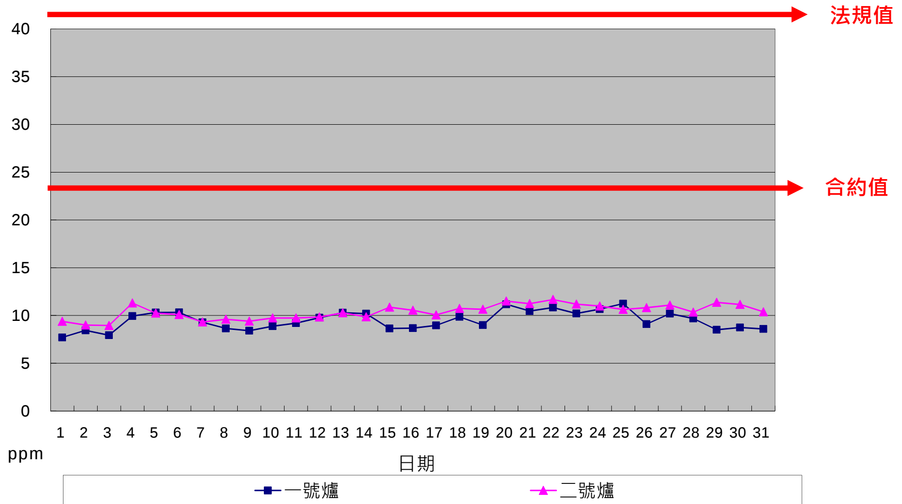
一百零八年一月份 HCl單日24小時整月排放監測紀錄
