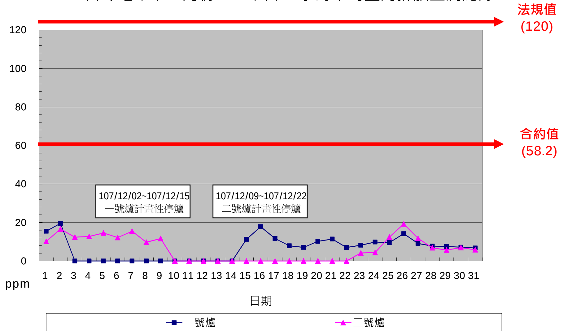
一百零七年十二月份 CO單日24小時平均整月排放監測紀錄
