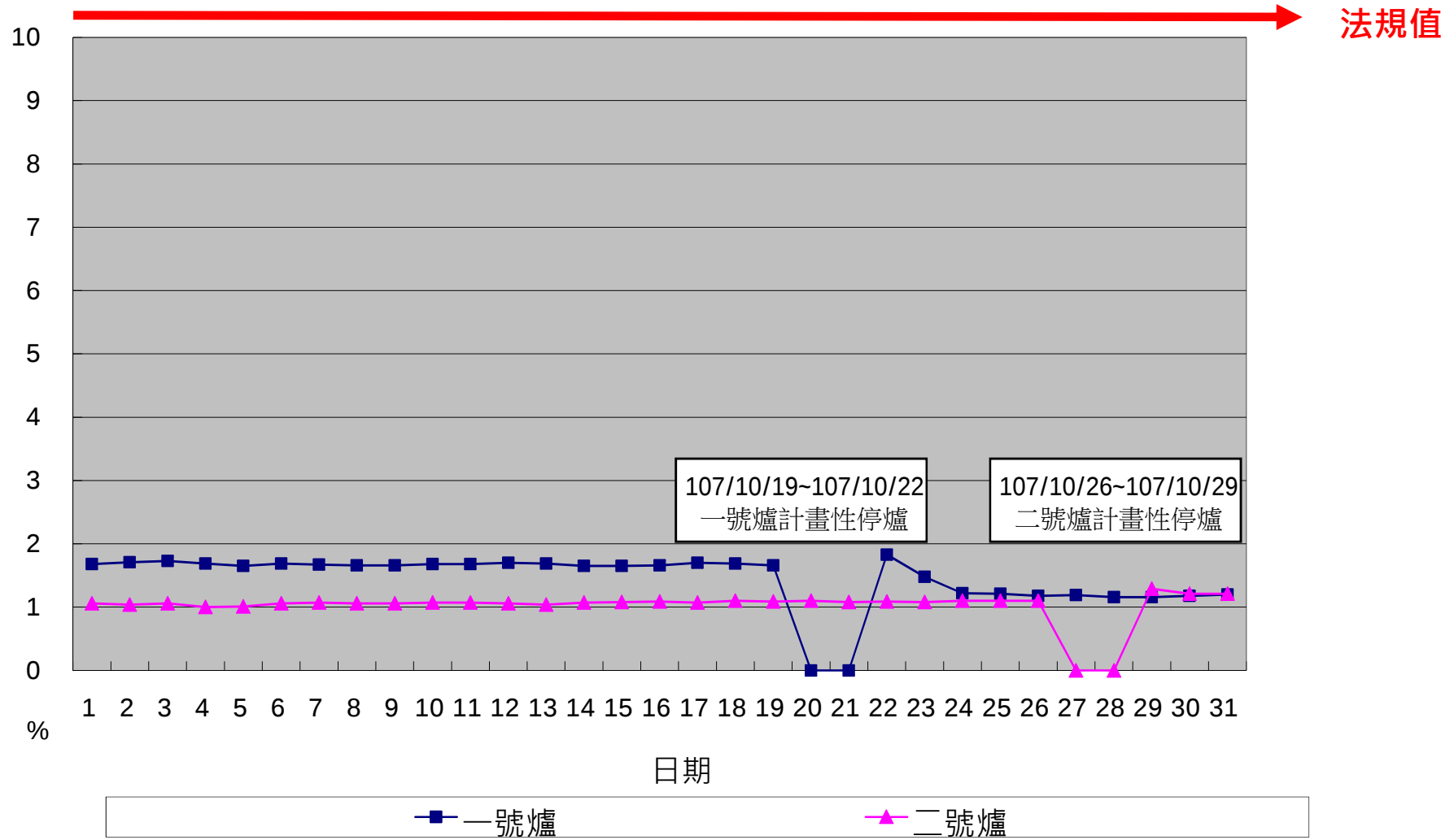
一百零七年十月份 OPACITY單日24小時整月排放監測紀錄
