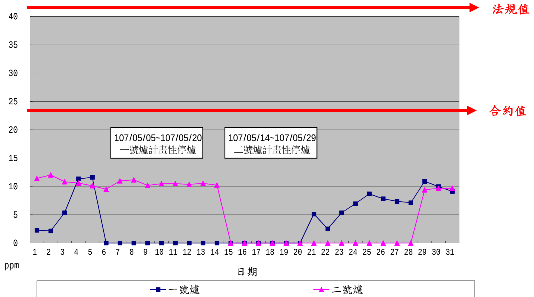
一百零七年五月份 HCl單日24小時整月排放監測紀錄
