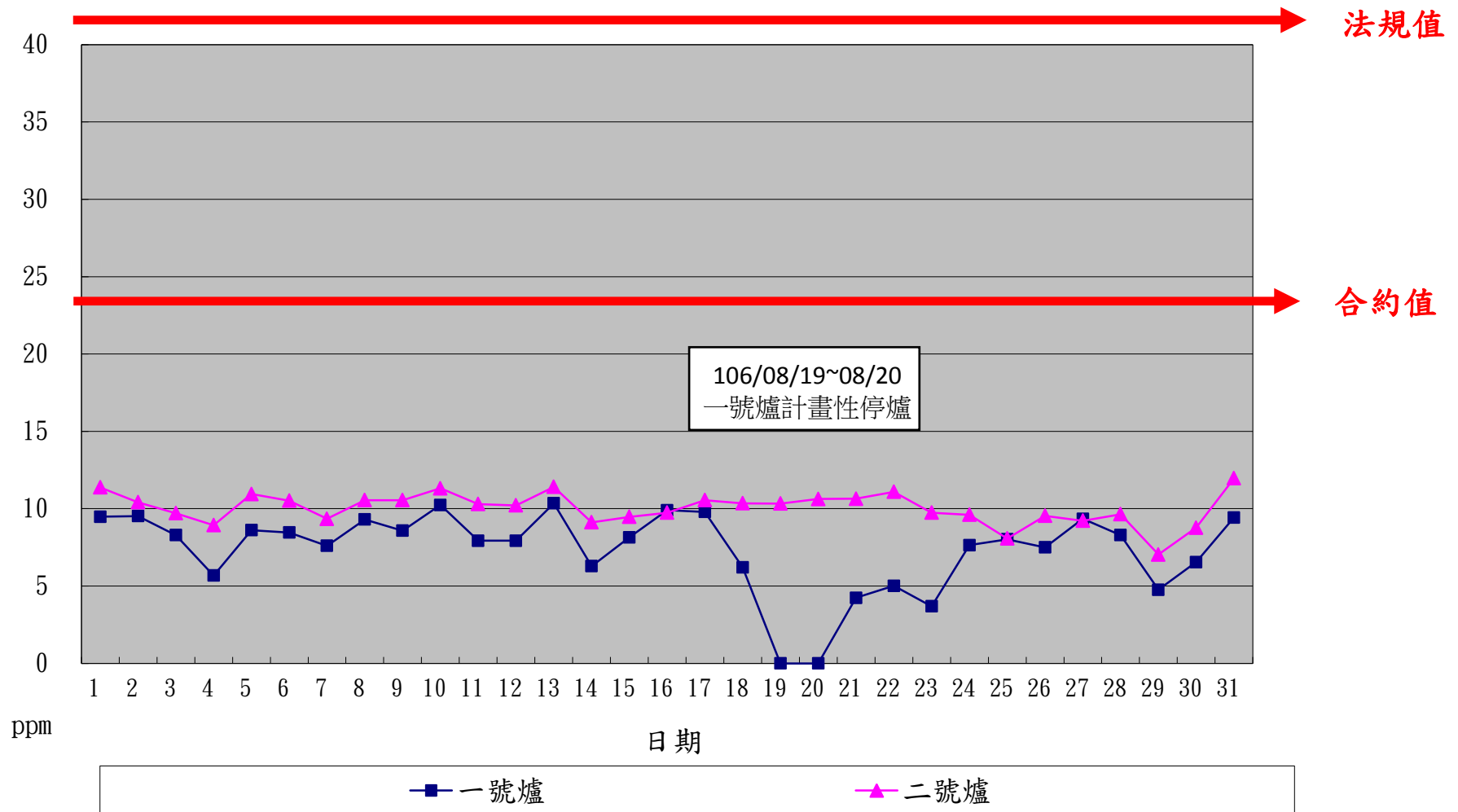
一百零六年八月份 HC1單日24小時整月排放監測紀錄
