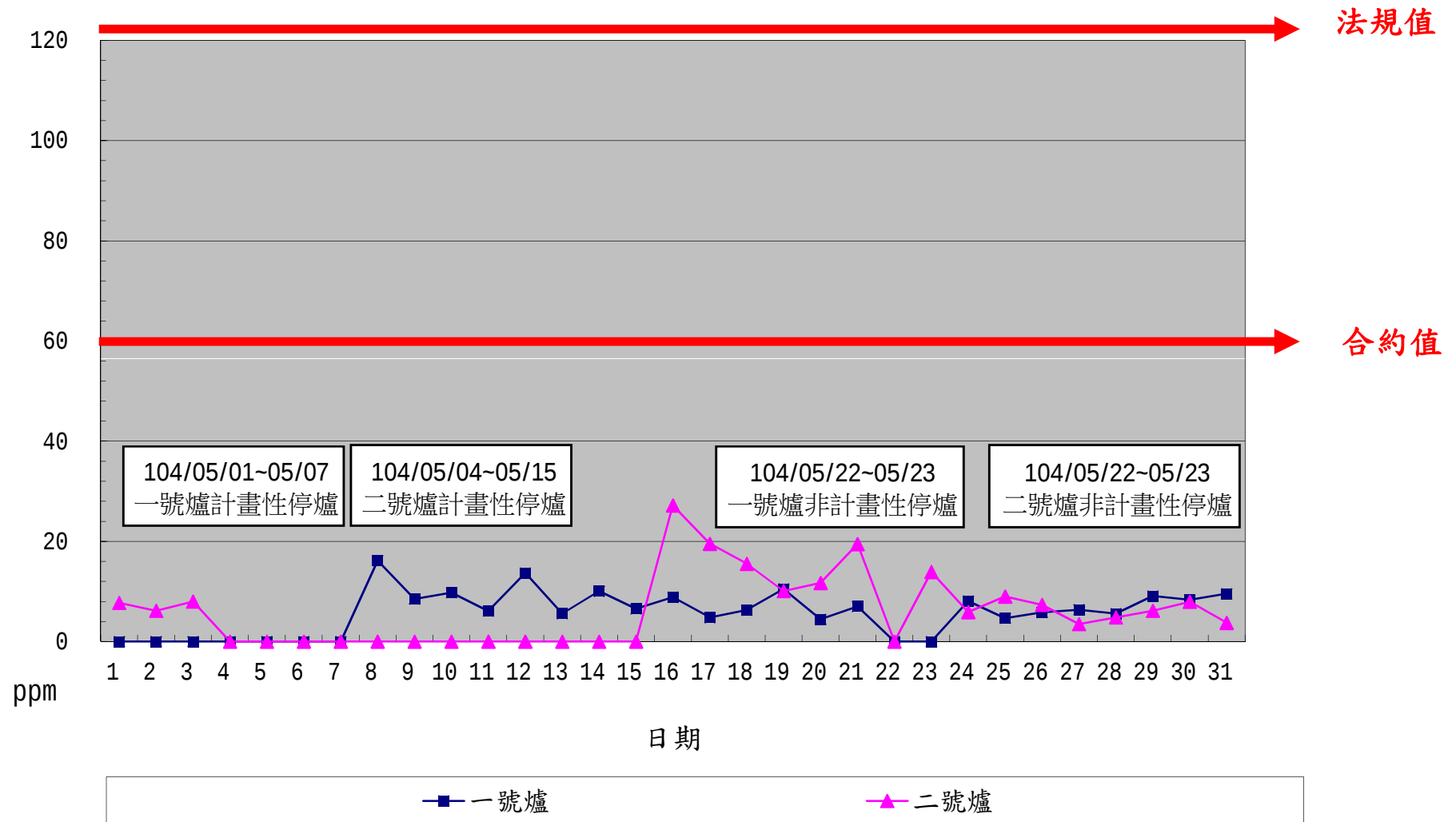
一百零四年五月份 CO單日24小時平均整月排放監測紀錄
